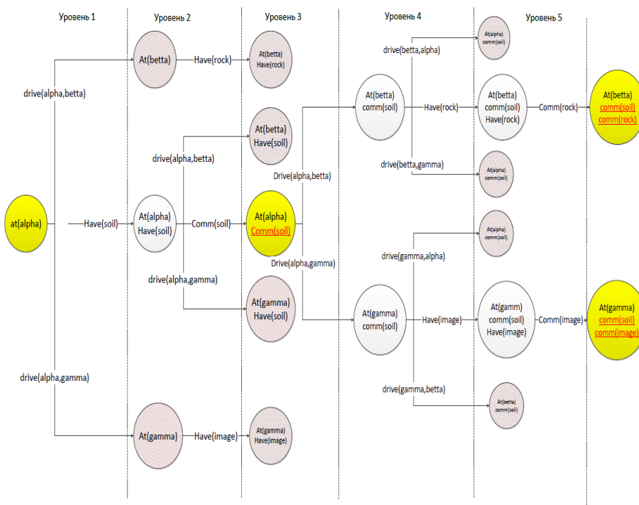
Рис. 3. Граф задачи о марсоходе
